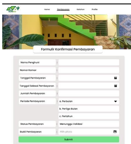
Gambar 6. Prototype Halaman Pembayaran Penghuni Kos
